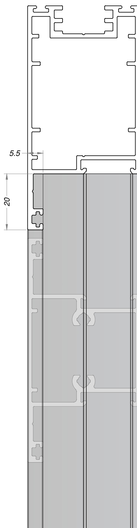
USINAGEM DE DESABE TRAVESSA
