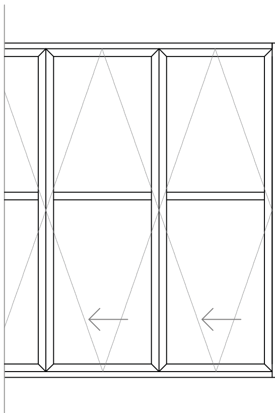
PORTA CAMARÃO "N" FOLHAS SEQUÊNCIAIS COM TRAVESSA E VIDRO
