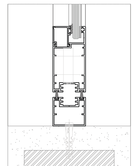
CORTE 04
