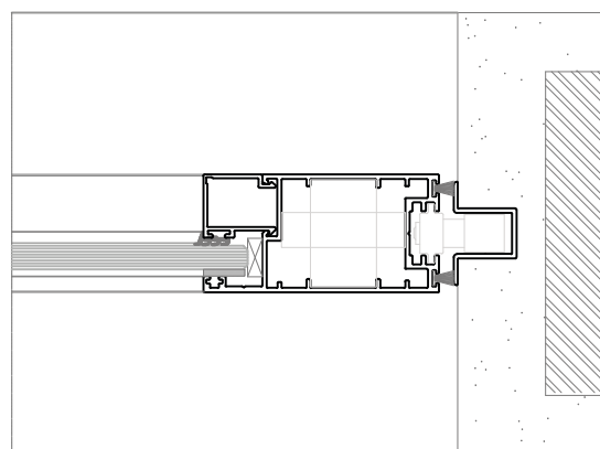
CORTE 01
