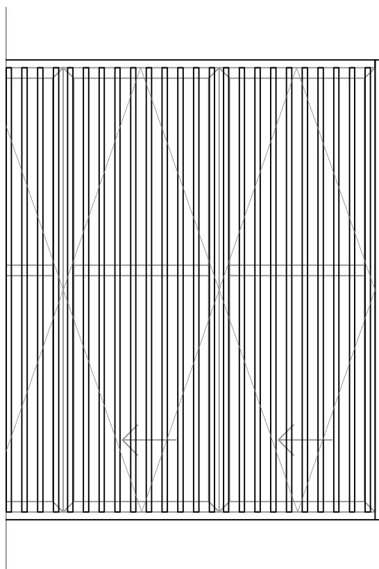
PORTA CAMARÃO "N" FOLHAS SEQUÊNCIAIS COM PREENCHIMENTO EXTERNO RIPADO OU MUXARABI COM TRAVESSA
