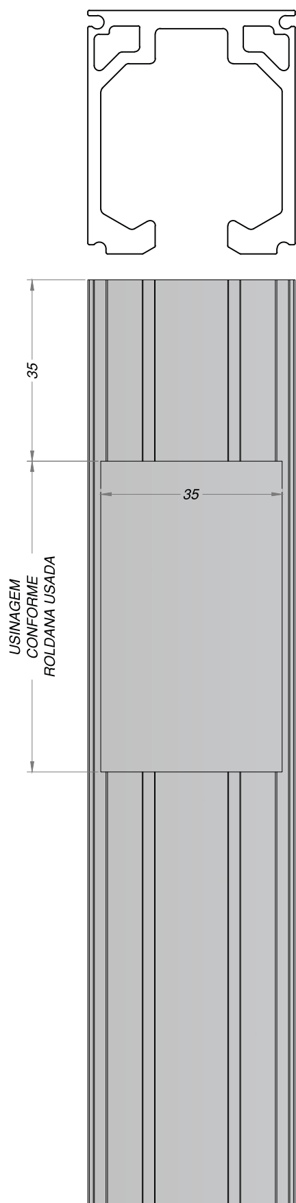
USINAGEM DE ENCAIXE DA ROLDANA
