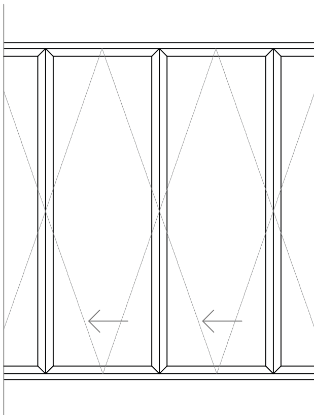
PORTA CAMARÃO "N" FOLHAS FECHAMENTO CENTRAL COM VIDRO
