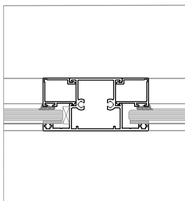
CORTE 02 LADO EXTERNO
