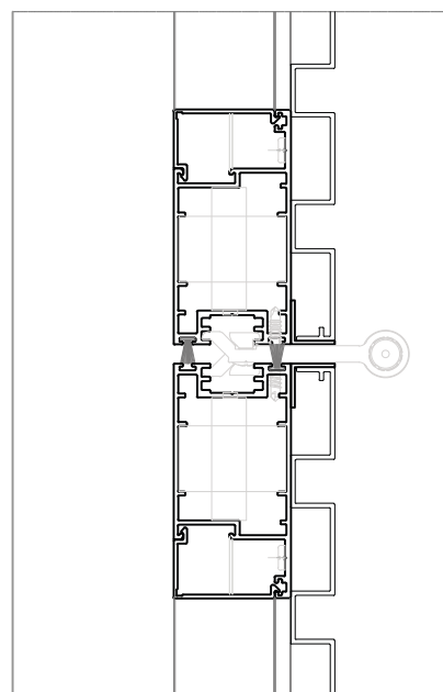
CORTE 05 LADO EXTERNO
