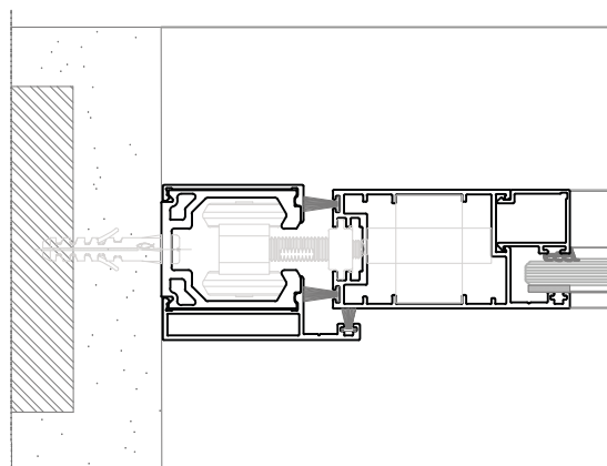
CORTE 03
