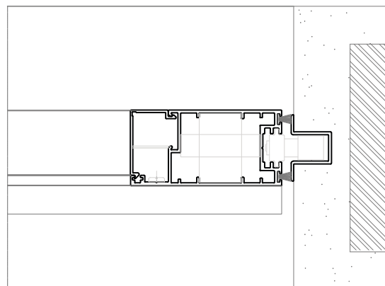
CORTE 01
