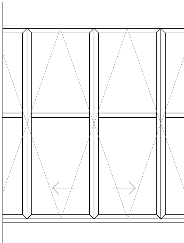
PORTA CAMARÃO "N" FOLHAS FECHAMENTO CENTRAL COM TRAVESSA E VIDRO
