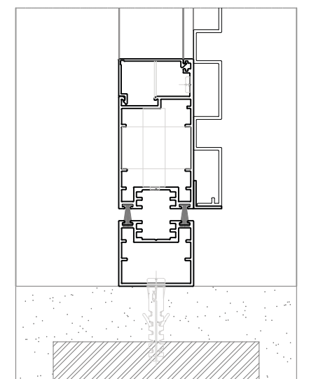
CORTE 04
