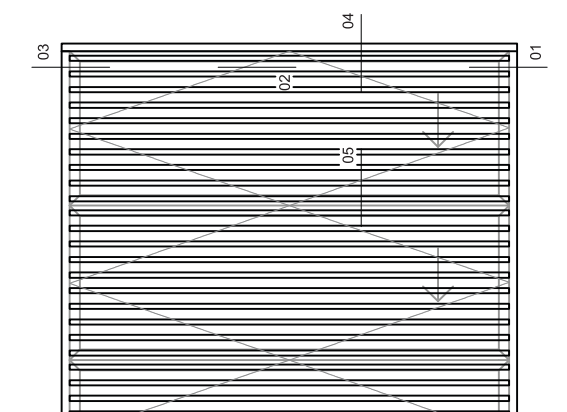
PORTA CAMARÃO COM RIPADO
