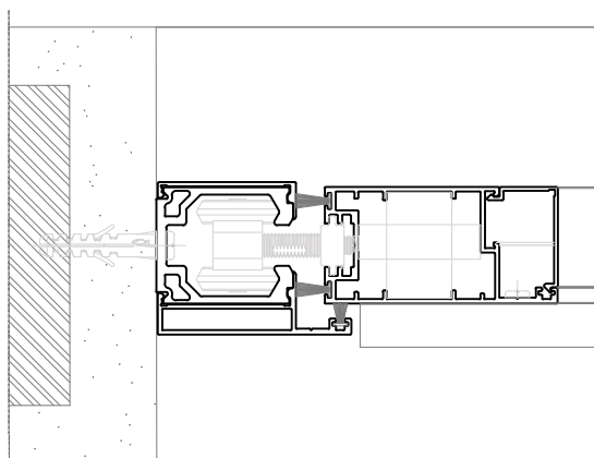
CORTE 03
